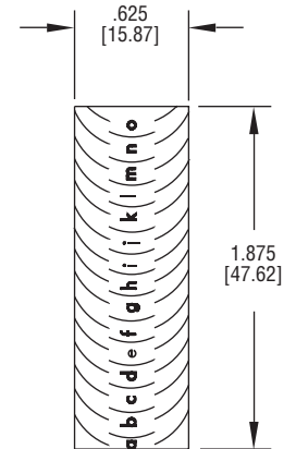
Trimmable Vane
