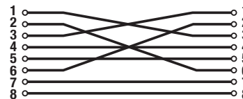
Câblage de croisement
