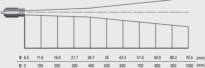
Optics CT LT SF, D:S = 15:1
