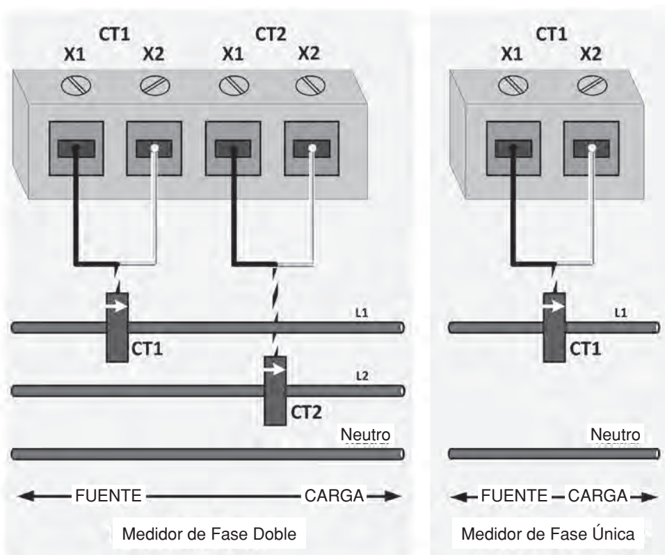
Figura 6 – Diagrama de Cableado del TC
