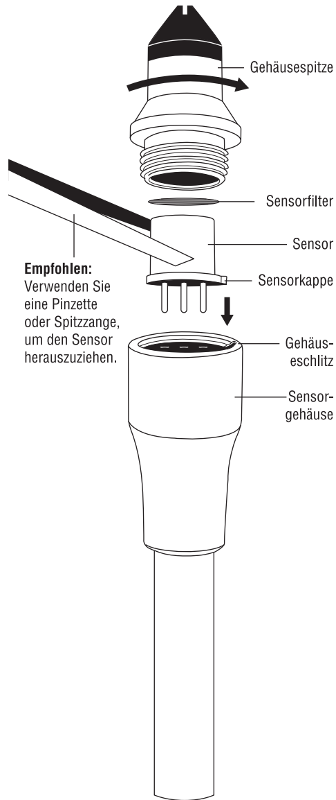
Abbildung: Sensoraustausch
