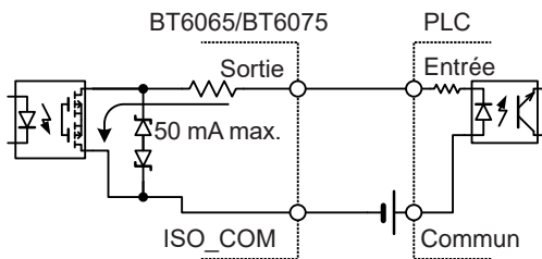
Raccordement à l'entrée PLC (commune positive)
