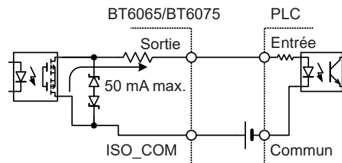
Raccordement à l'entrée PLC (commune négative)
