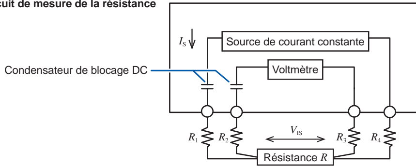
Circuit de mesure de la résistance
