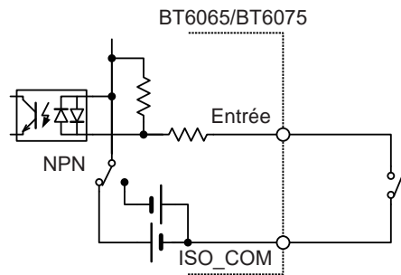
Raccordement au commutateur
