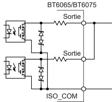
OR câblé
