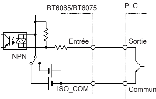
Raccordement à la sortie PLC (NPN)
