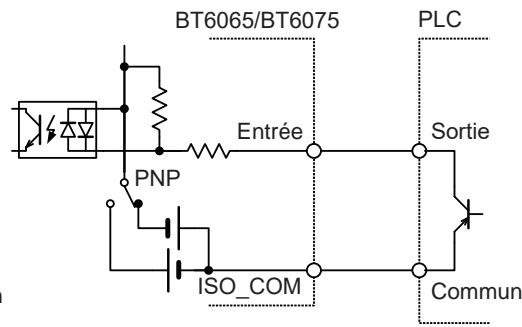
Raccordement à la sortie PLC (PNP)
