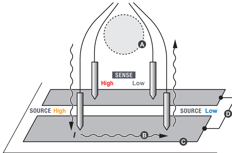
Dispositif spécialement conçu pour le réglage du zéro
