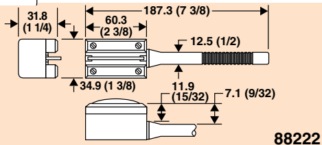
98221 Swivel 88221
