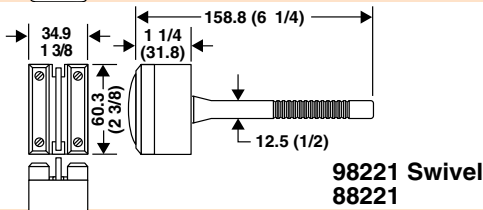
98220 Swivel 88220
