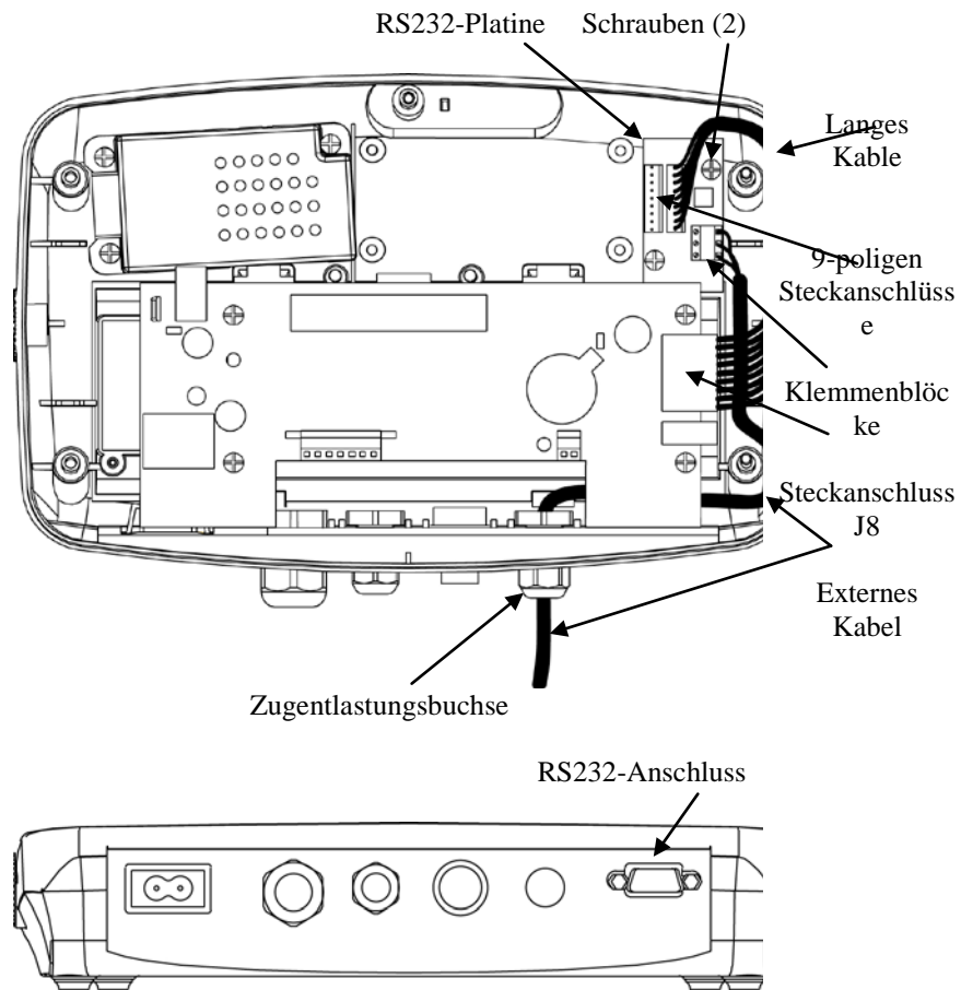
Abbildung 2.3. T51P, T71P
