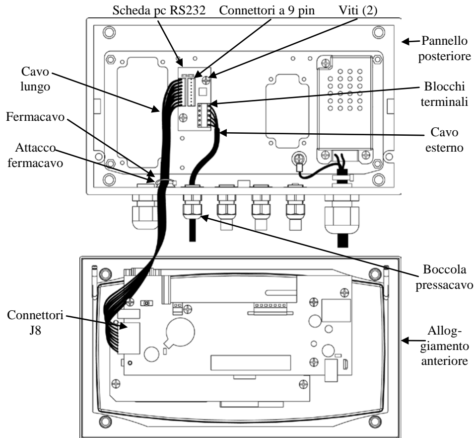
Figura 2.4. T51XW, T71XW
