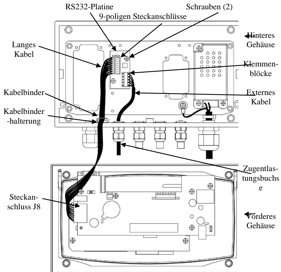
Abbildung 2.4. T51XW, T71XW
