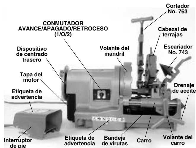
Figura 2 – Roscadora 1233
