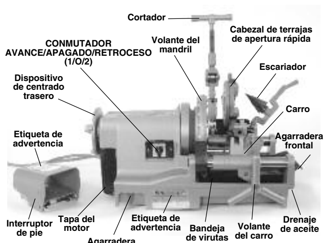
Figura 1 – Roscadora compacta 300
