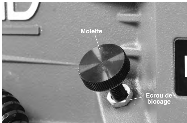
Figure 20 – Tendeur de courroie
