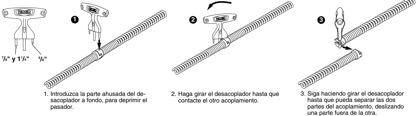
Figura 8 – Acoplamiento y desacoplamiento
