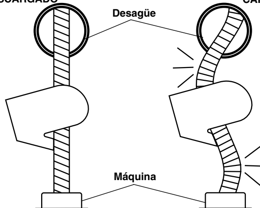
Figura 13 – Forma que adopta el cable cuando está descargado o cargado
