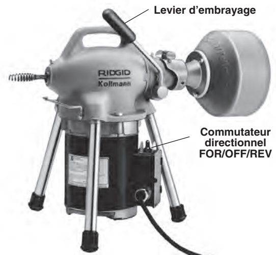
Figure 1 – Dégorgeoir K-50
