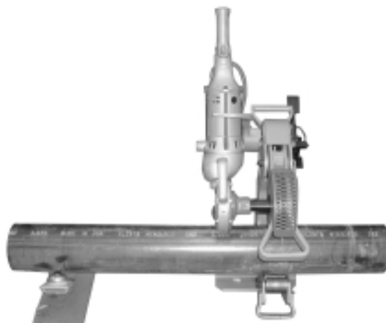
Figura 7C – Tubo corto a medianamente largo
