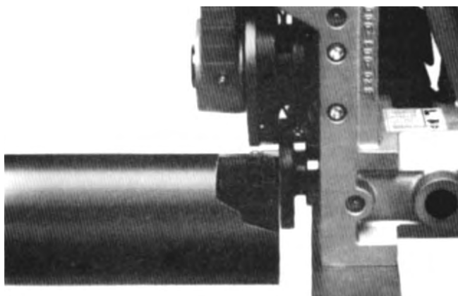
Figura 10 – Primer plano del tubo colocado contra el reborde del rodillo de accionamiento
