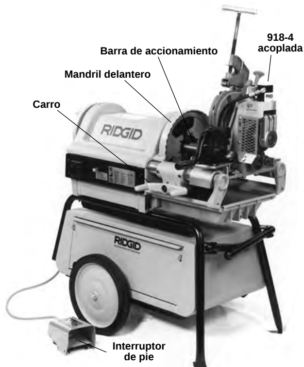
Figura 6 – Ranuradora a rodillos No. 918-4 montada a la Máquina Roscadora 1224
