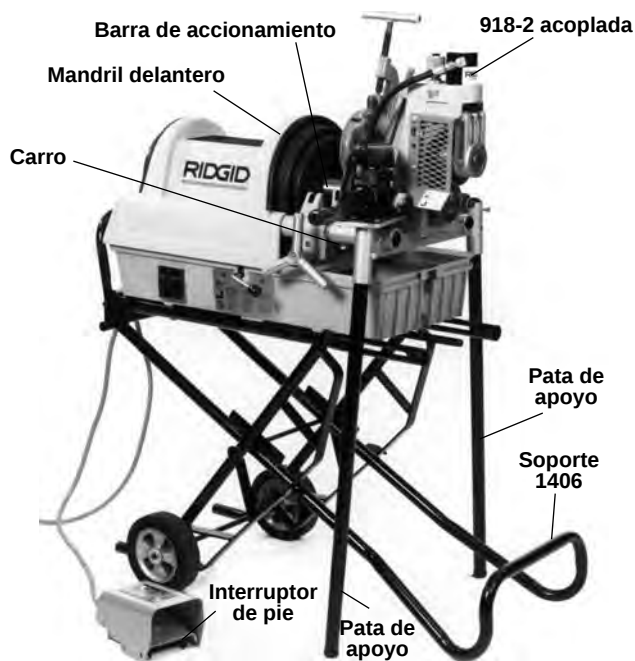
Figura 4 – La Ranuradora a Rodillos 918 montada a la Máquina Roscadora 1822 sobre el Soporte 1406
