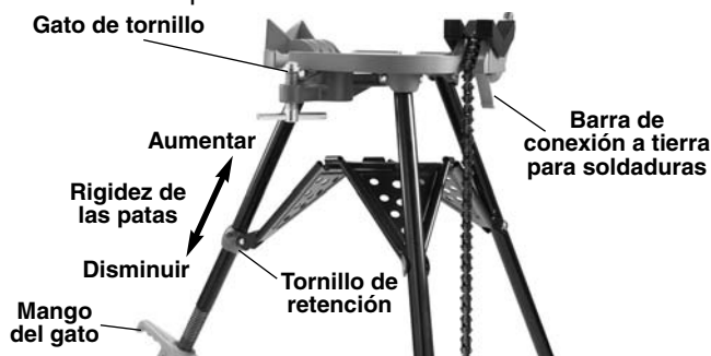
Figura 2 – Ajuste de la tensión de las patas del trípode (460-12)
