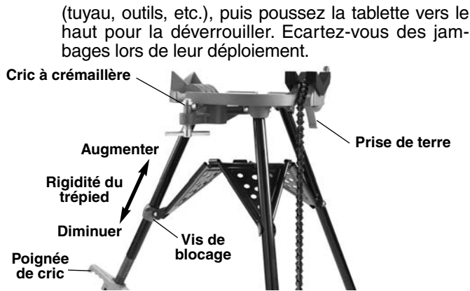
Figure 2 – Réglage de la tablette (460-12)
