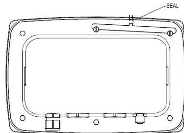
Abbildung 7-2. TD52XW Drahtversiegelung
