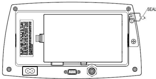
Abbildung 7-1. TD52P Drahtversiegelung
