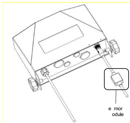
Abbildung 7-5. Anschlusskabel mit Stecker und Speicher-Modul
