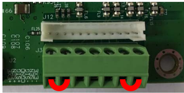
Abbildung 2-4 Jumperverbindungen
