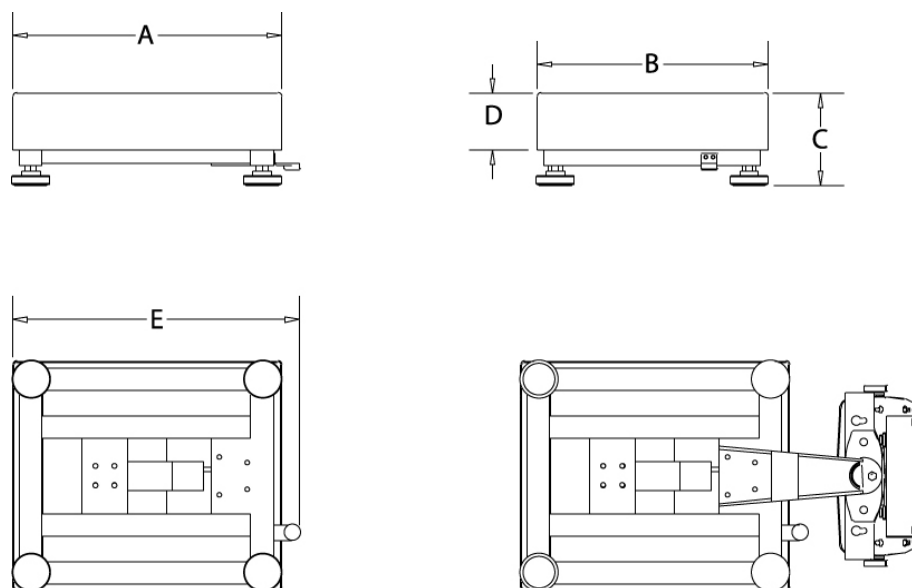
Figure 1. Schéma des dimensions de la plate-forme Defender.
