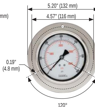
40-911 Front Flange
