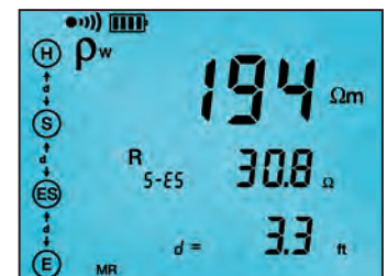
Wenner Test
