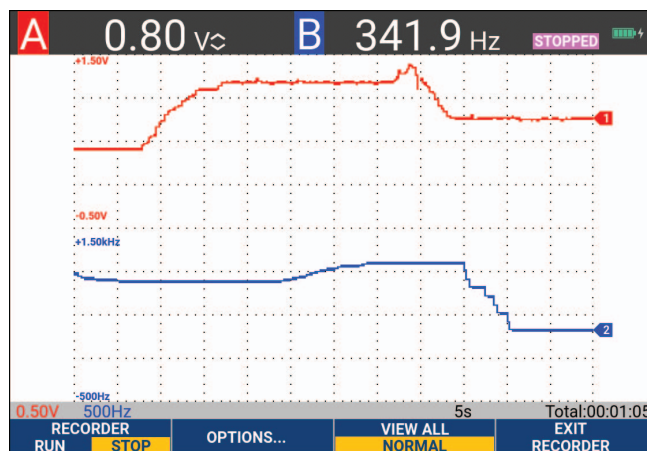
Figure 17. Relevé TrendPlot
