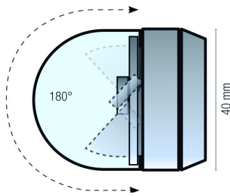
Fig. 4: Tilts 180°
